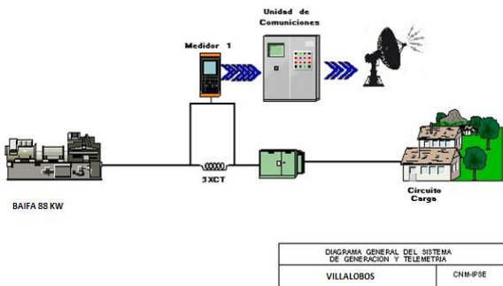
Ilustración 34: Esquema de conexión de la localidad
