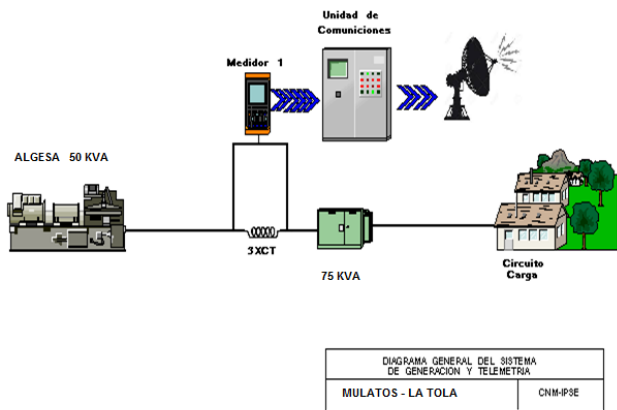
Ilustración 192: Esquema de conexión de la localidad
