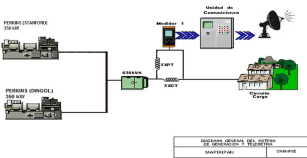
Ilustración 165: Esquema de conexión de la localidad
