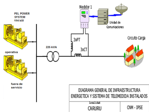
Ilustración 207: Esquema de conexión de la localidad
