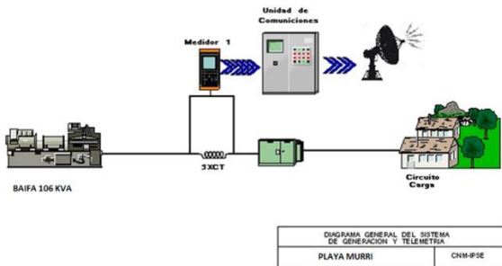
Ilustración 4: Esquema de conexión de la localidad
