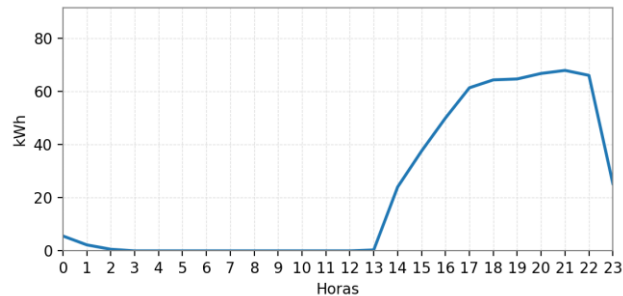
Ilustración 117: Curva de Carga Promedio Diaria Mensual.
