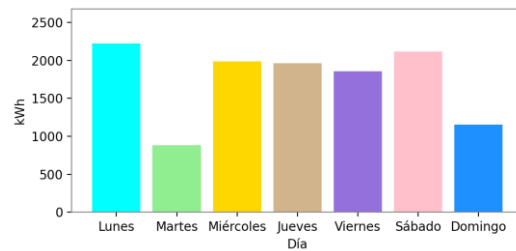
Ilustración 199: Energía entregada por día de la semana.
