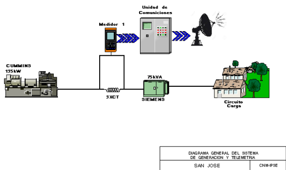
Ilustración 55: Esquema de conexión de la localidad
