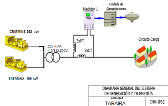
Ilustración 213: Esquema de conexión de la localidad
