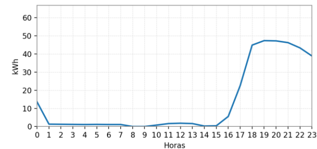
Ilustración 197: Curva de Carga Promedio Diaria Mensual.
