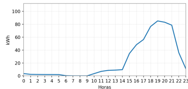
Ilustración 30: Curva de Carga Promedio Diaria Mensual.
