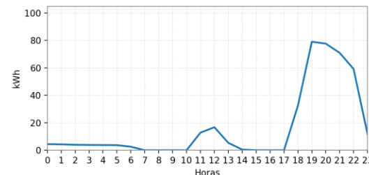
Ilustración 200: Curva de Carga Promedio Diaria Mensual.
