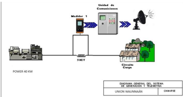
Ilustración 138: Esquema de conexión de la localidad
