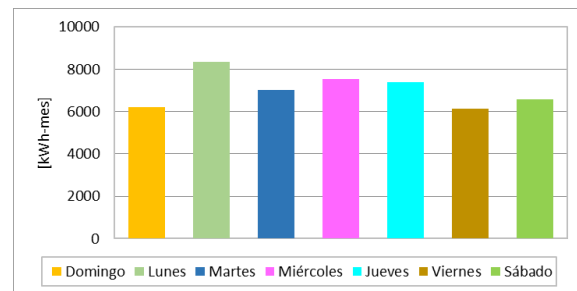
Ilustración 157: Energía entregada por día de la semana.
