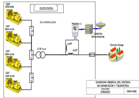
Ilustración 91: Esquema de conexión de la localidad
