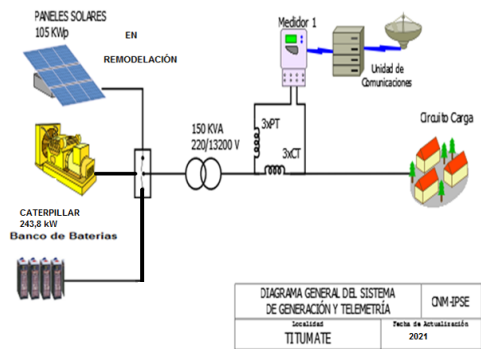
Ilustración 129: Esquema de conexión de la localidad
