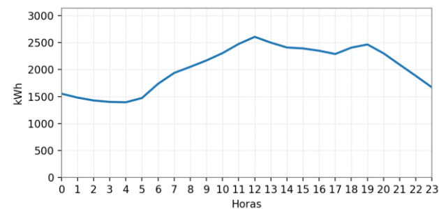
Ilustración 212: Curva de Carga Promedio Diaria Mensual.
