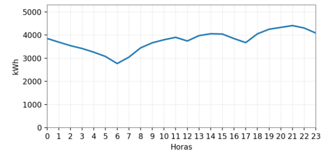
Ilustración 218: Curva de Carga Promedio Diaria Mensual.
