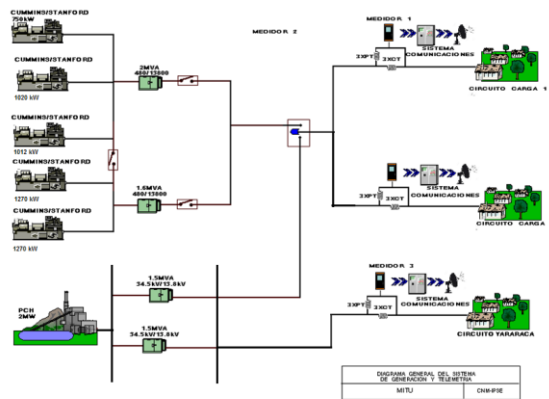
Ilustración 210: Esquema de conexión de la localidad
