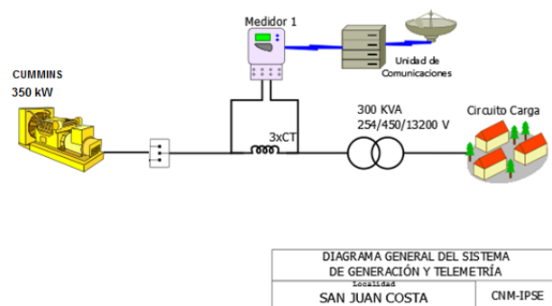
Ilustración 198: Esquema de conexión de la localidad
