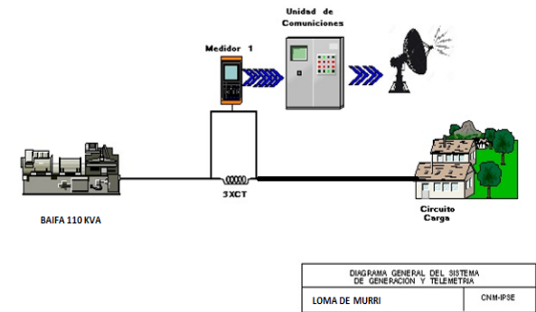
Ilustración 7: Esquema de conexión de la localidad
