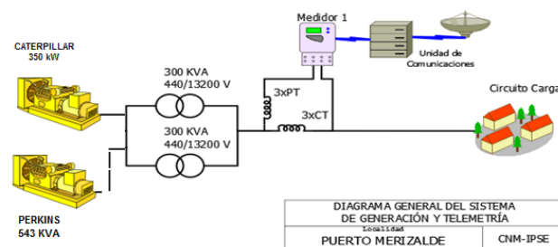
Ilustración 201: Esquema de conexión de la localidad
