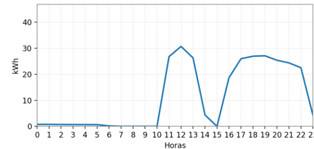
Ilustración 188: Curva de Carga Promedio Diaria Mensual.
