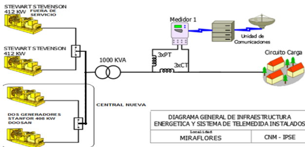
Ilustración 153: Esquema de conexión de la localidad
