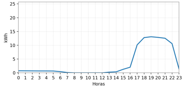
Ilustración 179: Curva de Carga Promedio Diaria Mensual.
