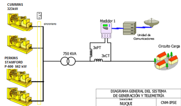
Ilustración 97: Esquema de conexión de la localidad
