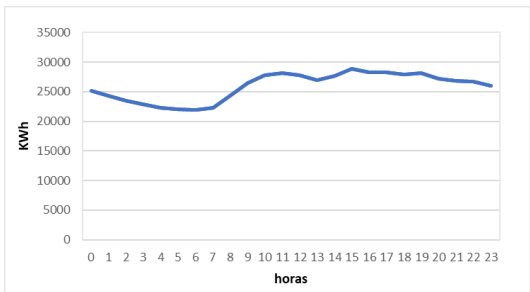
Ilustración 15: Curva de Carga Promedio Diaria Mensual.
