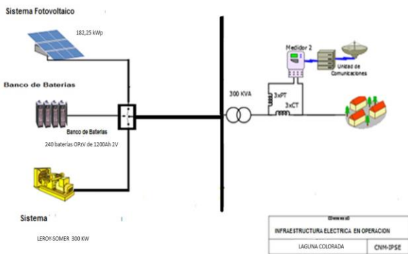
Ilustración 150: Esquema de conexión de la localidad
