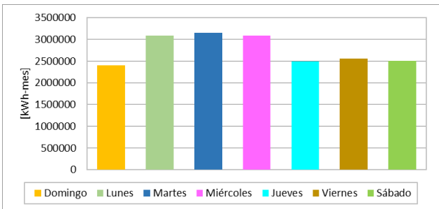
Ilustración 14: Energía entregada por día de la semana.
