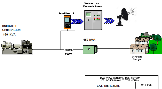
Ilustración 189: Esquema de conexión de la localidad
