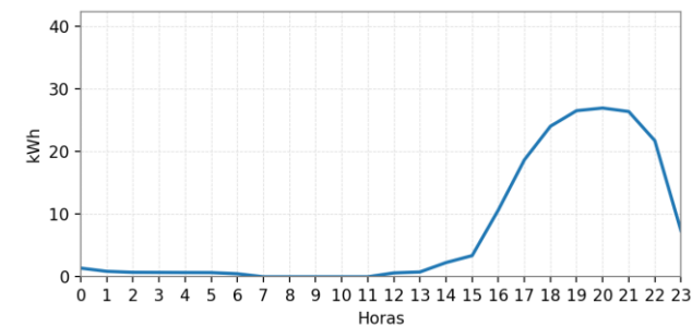
Ilustración 182: Curva de Carga Promedio Diaria Mensual.
