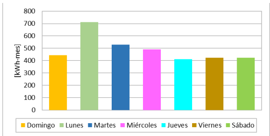
Ilustración 104: Energía entregada por día de la semana.
