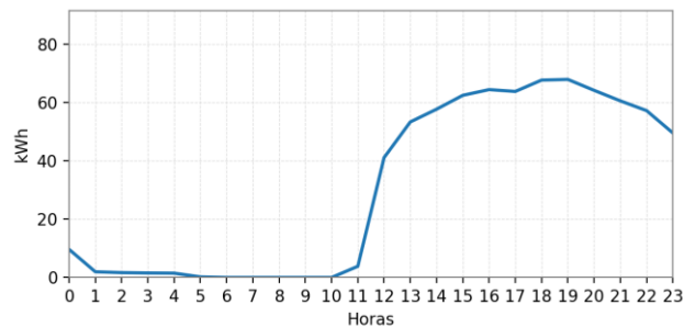
Ilustración 209: Curva de Carga Promedio Diaria Mensual.
