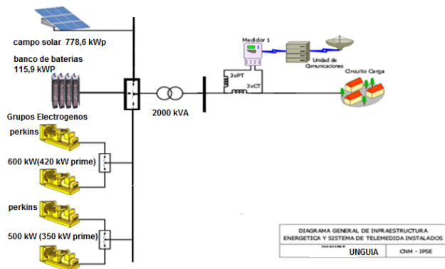
Ilustración 132: Esquema de conexión de la localidad
