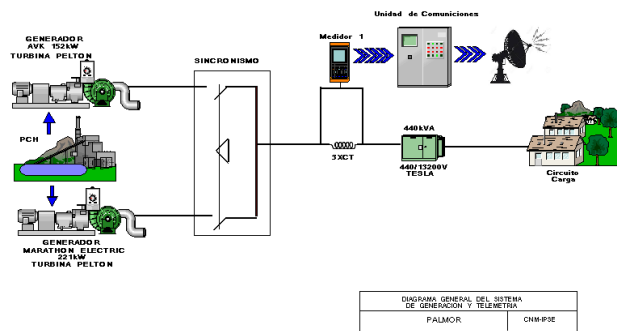
Ilustración 162: Esquema de conexión de la localidad
