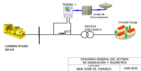
Ilustración 195: Esquema de conexión de la localidad
