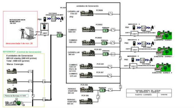
Ilustración 216: Esquema de conexión de la localidad
