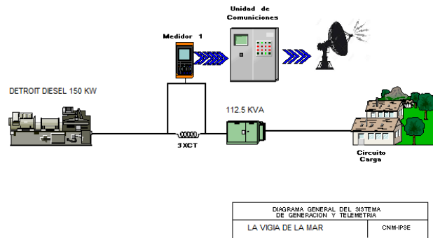
Ilustración 186: Esquema de conexión de la localidad
