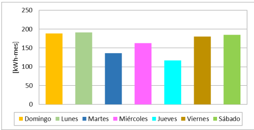
Ilustración 89: Energía entregada por día de la semana.
