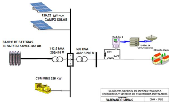
Ilustración 144: Esquema de conexión de la localidad
