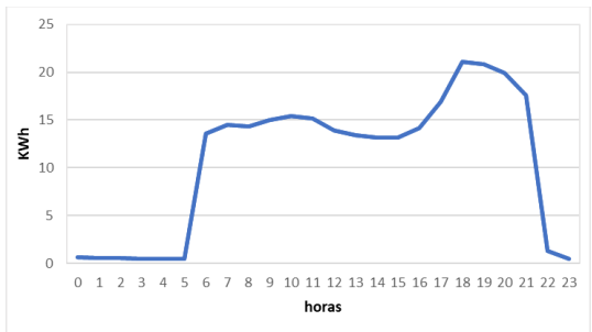
Ilustración 152: Curva de Carga Promedio Diaria Mensual.
