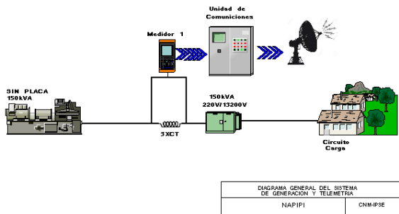
Ilustración 94: Esquema de conexión de la localidad
