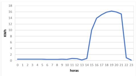
Ilustración 105: Curva de Carga Promedio Diaria Mensual.
