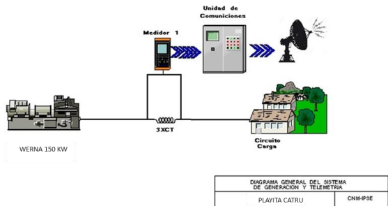
Ilustración 109: Esquema de conexión de la localidad
