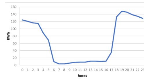
Ilustración 158: Curva de Carga Promedio Diaria Mensual.
