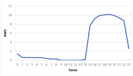
Ilustración 114: Curva de Carga Promedio Diaria Mensual.
