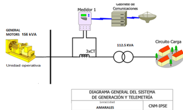
Ilustración 171: Esquema de conexión de la localidad
