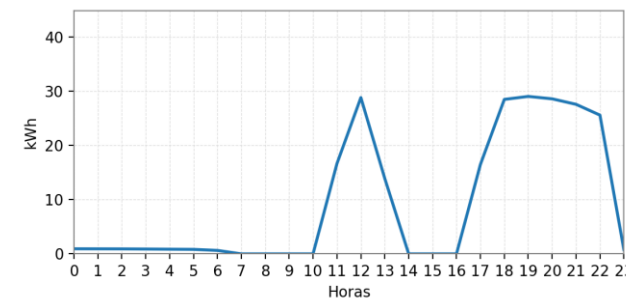
Ilustración 206: Curva de Carga Promedio Diaria Mensual.
