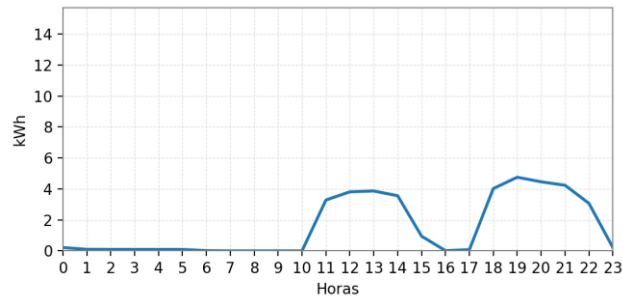
Ilustración 102: Curva de Carga Promedio Diaria Mensual.
