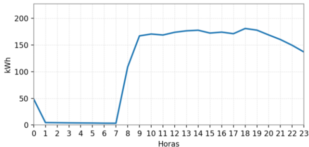
Ilustración 146: Curva de Carga Promedio Diaria Mensual.
