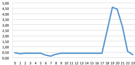
Ilustración 6: Curva de Carga Promedio Diaria Mensual.
