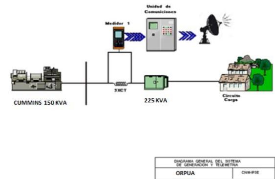
Ilustración 100: Esquema de conexión de la localidad
