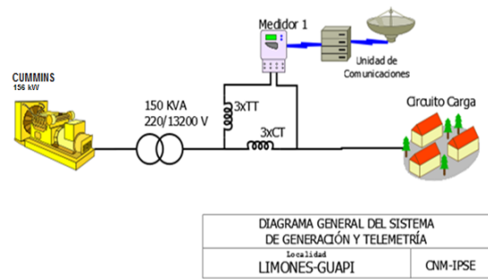
Ilustración 43: Esquema de conexión de la localidad
