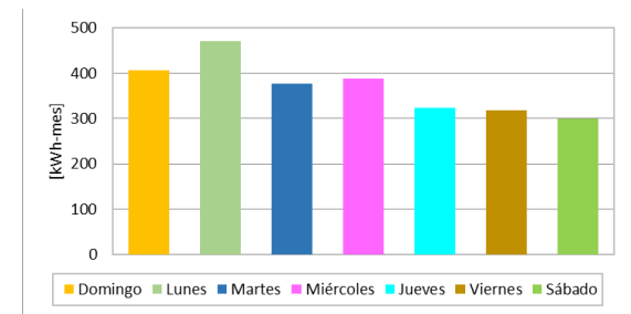
Ilustración 113: Energía entregada por día de la semana.
