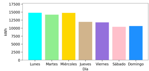
Ilustración 121: Energía entregada por día de la semana.
