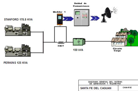
Ilustración 31: Esquema de conexión de la localidad
