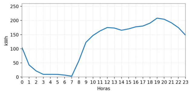
Ilustración 122: Curva de Carga Promedio Diaria Mensual.
