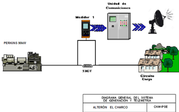
Ilustración 168: Esquema de conexión de la localidad
