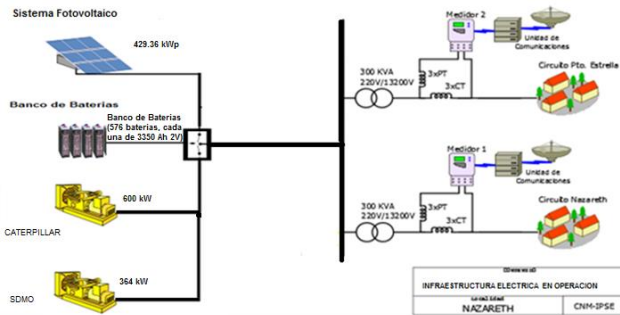
Ilustración 159: Esquema de conexión de la localidad
