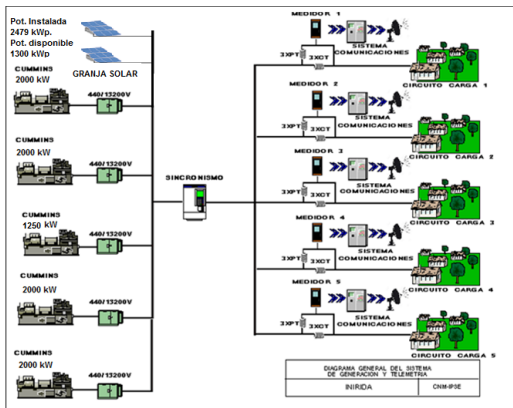
Ilustración 147: Esquema de conexión de la localidad
