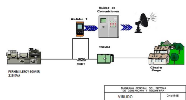
Ilustración 141: Esquema de conexión de la localidad
