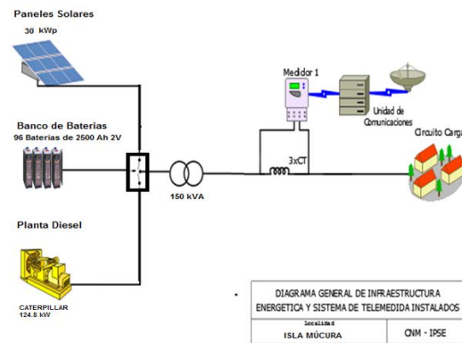
Ilustración 19: Esquema de conexión de la localidad
