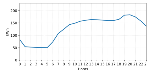
Ilustración 203: Curva de Carga Promedio Diaria Mensual.
