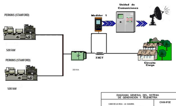
Ilustración 156: Esquema de conexión de la localidad
